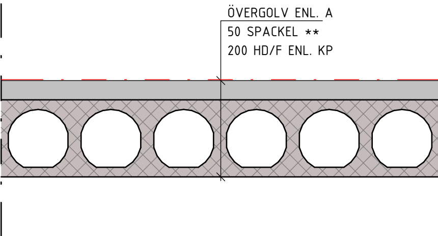
BJL01 1 : 10 ** MED LOKALA FALL MOT BRUNNAR
