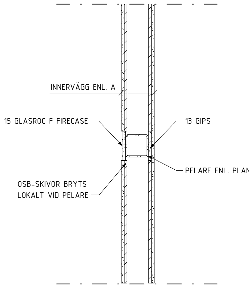
PRINCIPDETALJ 1:10 BRANDSKYDD AV PELARE I VÄGG ÖVRIGT
