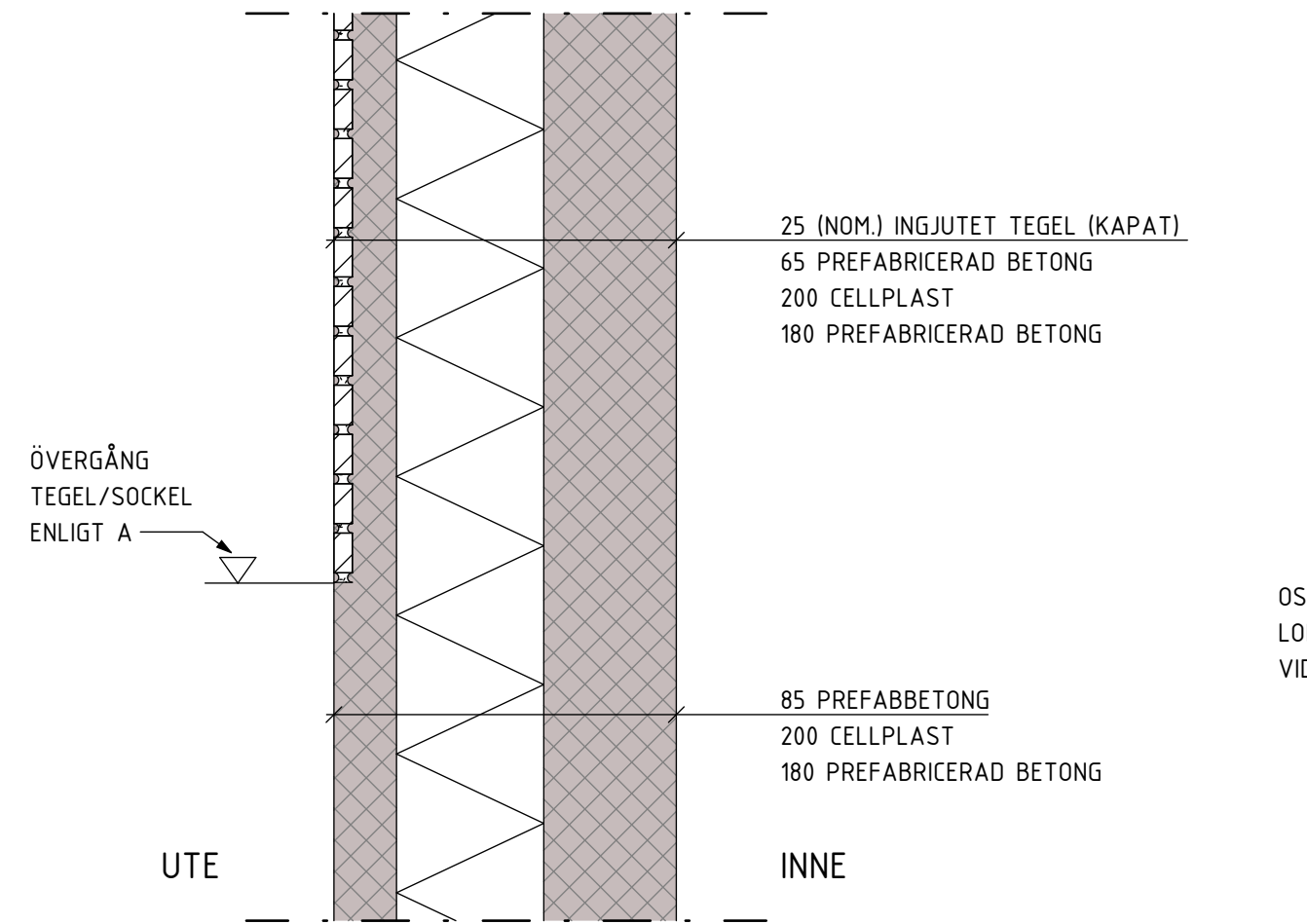
YVB01 1 : 10 YTTERVÄGG
