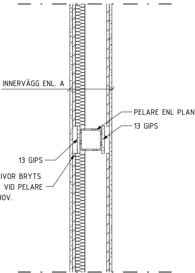
PRINCIPDETALJ 1:10 BRANDSKYDD AV PELARE I VÄGG MOT VAGNHALL
